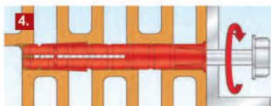
4. Заворачивание шурупа
