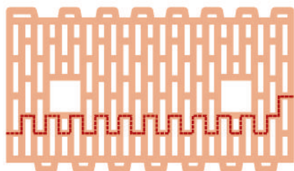
Рис. 5. Теплопередача через керамические стенки
